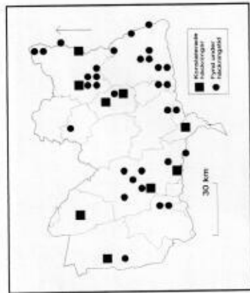
Figur 16. Konstaterade häckningar och övriga fynd under häckningstid av rödbena i Västmanland 1984-93, fördelat på 5x5 km-rutor.
