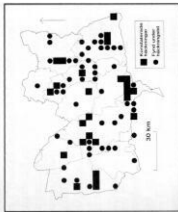
Figur 15. Konstaterade häckningar och övriga fynd under häckningstid av tornfalk i Västmanland 1982-93, fördelat på 5x5 km-rutor.
