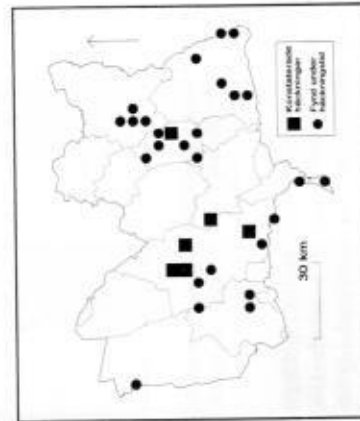
Figur 4. Konstaterade häckningar och övriga fynd under häckningstid av blåsand i Västmanland 1982-93, fördelat på 5x5 km-rutor.
