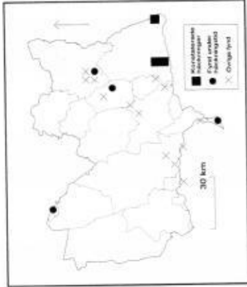
Figur 5. Konstaterade häckningar, fynd under häckningstid samt övriga fynd av snatterand i Västmanland 1982-93, fördelat på 5x5 km-rutor.
