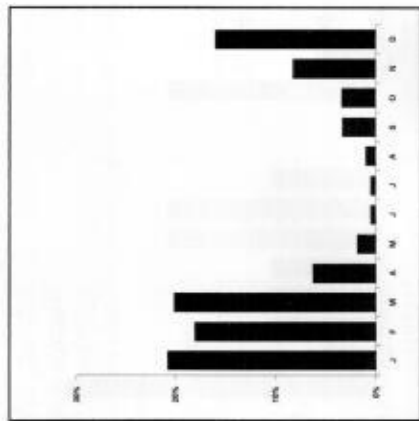
Figur 14. Fågeldagar av havsörn i Västmanland 1982-93, procentuell fördelning på årets månader.
