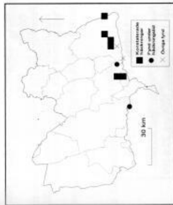
Figur 18. Konstaterade häckningar, fynd under häckningstid samt övriga fynd av pungmues i Västmanland 1982-93, fördelat på 5x5 km-rutor. Det bör noteras att samliga fynd härifrån från femårsperioden 1989-93 och att byggande hantverksarbetare anses som konstaterad häckning.
