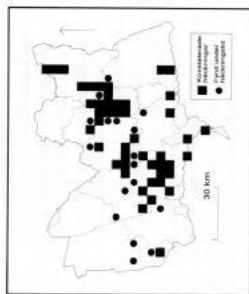
Figur 3. Konstaterade häckningar och övriga fynd under häckningsåret av sångsvan i Västmanland 1982-93, fördelat på 5x5 km-rutor.
