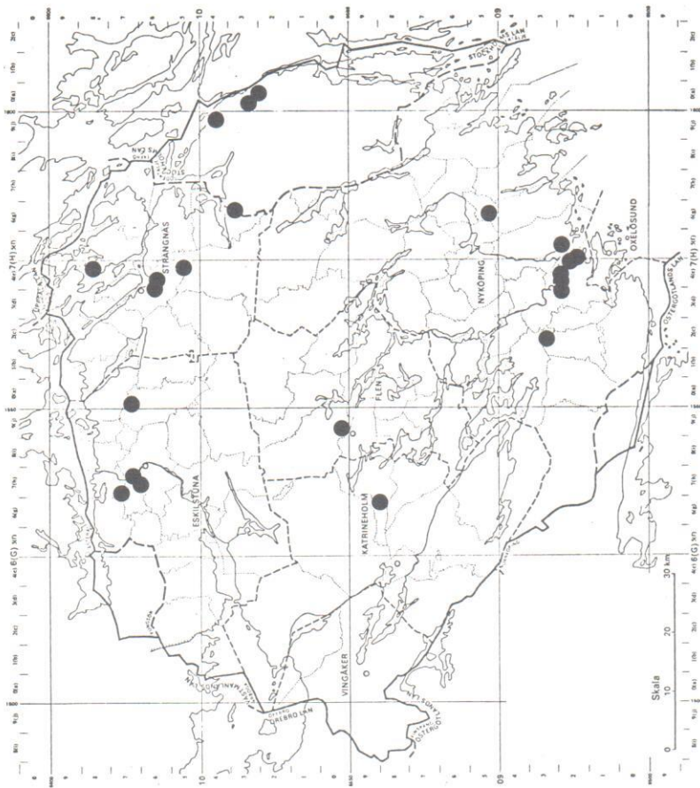
Figur 2. Karta över rapporterade häckningslokaler för mindre strandpipare 1975-80. (Map of reported breeding localities of Little Ringed Plover, Charadrius dubius , 1975-80.)
